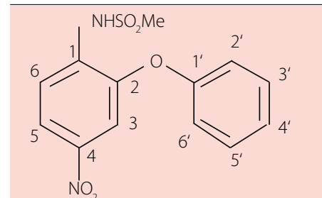
Obrázek 1. 4-nitro-2-phenoxy-methane-sulphonanilide
